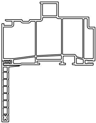
2" FLUSH FIN
